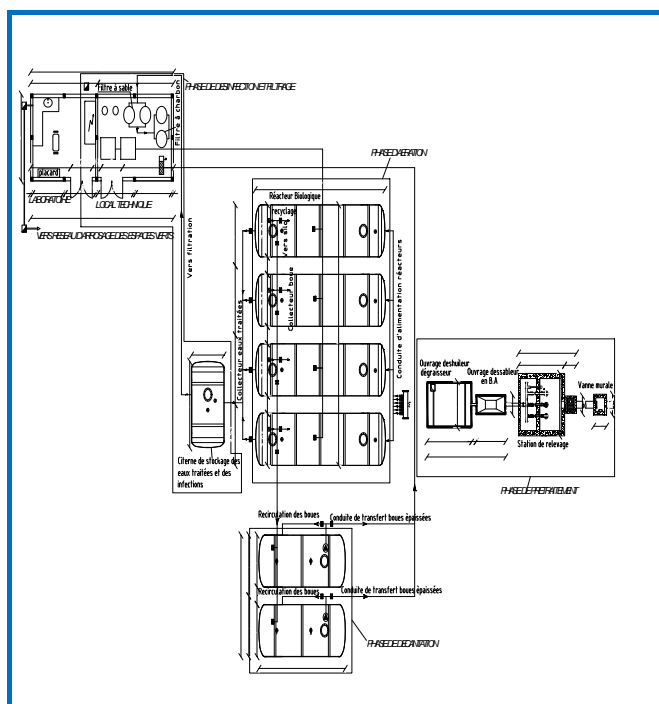
Mini Station d'épuration
